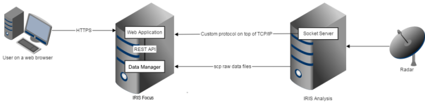
Figura 7 Caminhos de fornecimento de dados de radar
