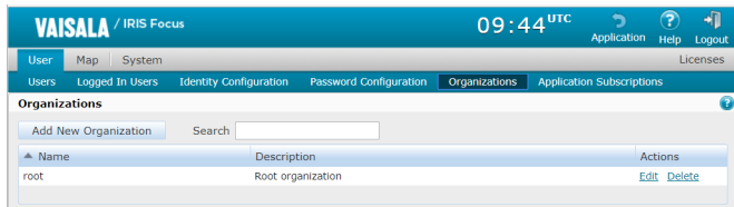
Рис. 60 Представление Организации
