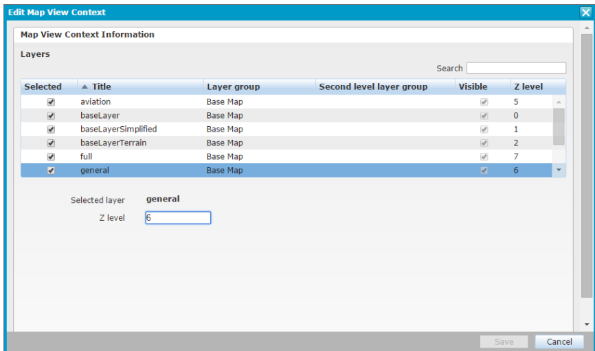
Рис. 62 Изменение содержимого карт
