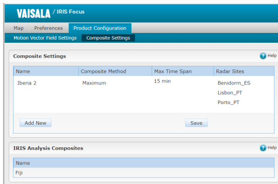
Рис. 63 Настройки композиции
