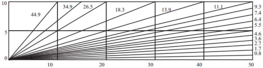
Figure 23 Exemple de balayage volumétrique à 15 inclinaisons
