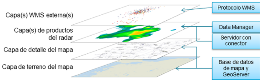
Figura 4 Capas de los productos de IRIS Focus
