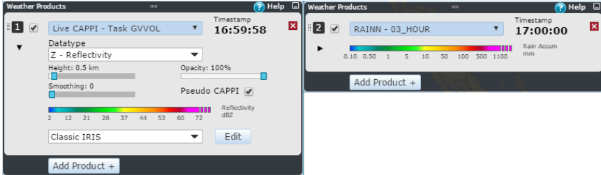
Figura 6 Configuración del producto a pedido y de IRIS Analysis
