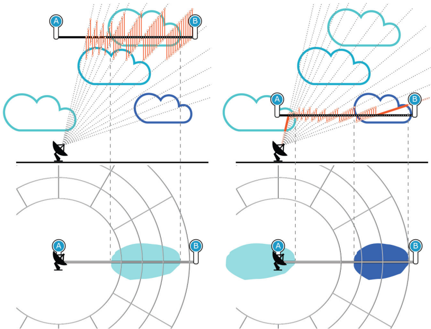
Figura 37 Extensión de Pseudo CAPPI a CAPPI
