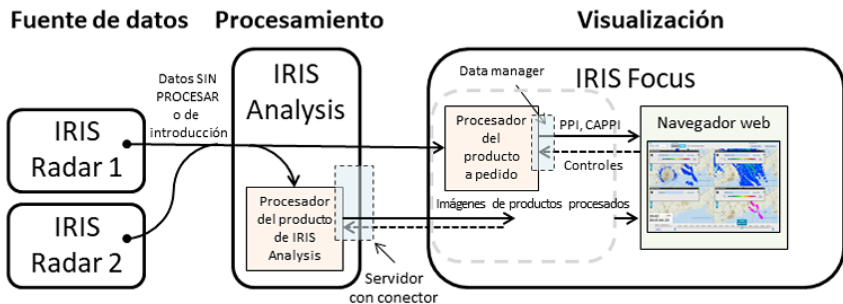
Figura 26 Flujo de datos de IRIS Focus
