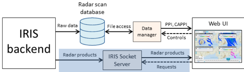
Figura 51 Flujo de datos del producto de IRIS Analysis a IRIS Focus
