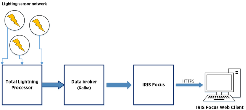
Figura 12 Arquitectura de relámpagos de IRIS Focus
