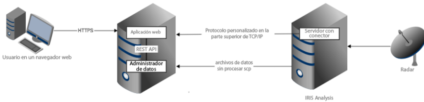
Figura 17 Rutas de entrega de los datos del radar
