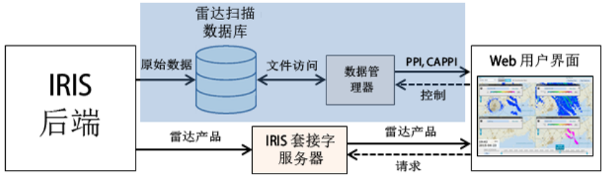
图 8 按需产品组件
