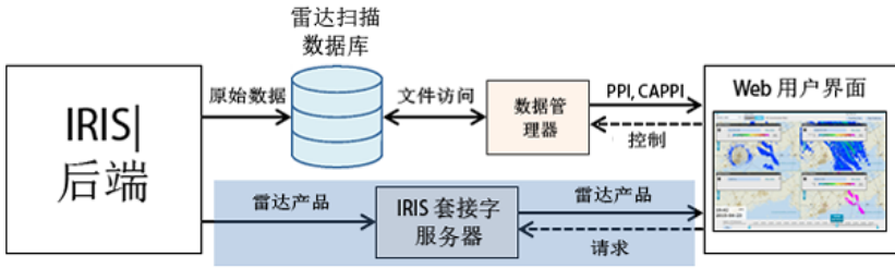
图 10 IRIS Analysis 到 IRIS Focus 的产品数据流
