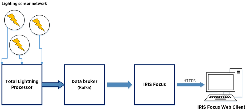
图 12 IRIS Focus 闪电体系结构
