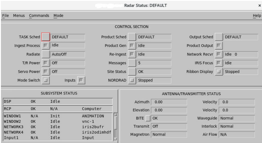
图 20 IRIS Radar 状态菜单
