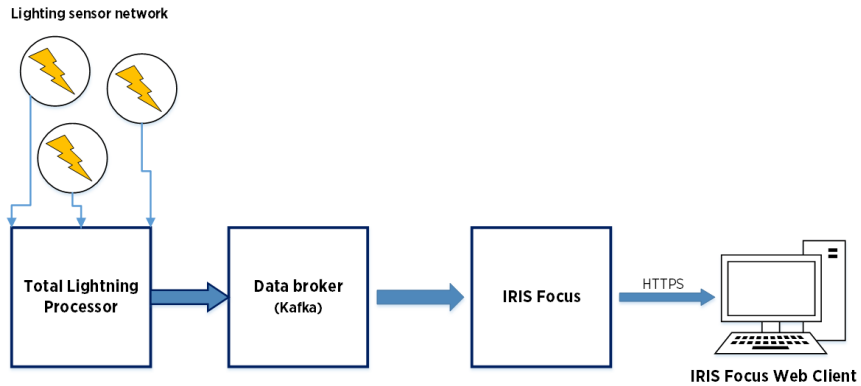
Figura 53 Arquitectura de relámpagos de IRIS Focus
