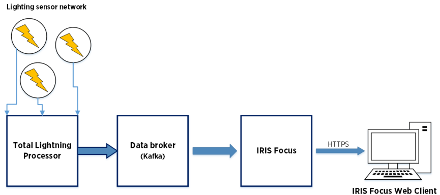
Рис. 53 Архитектура молний IRIS Focus
