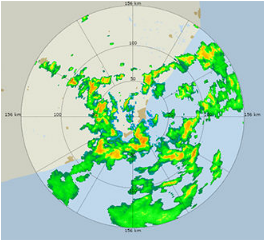
图 27 降水中的信号反射率
