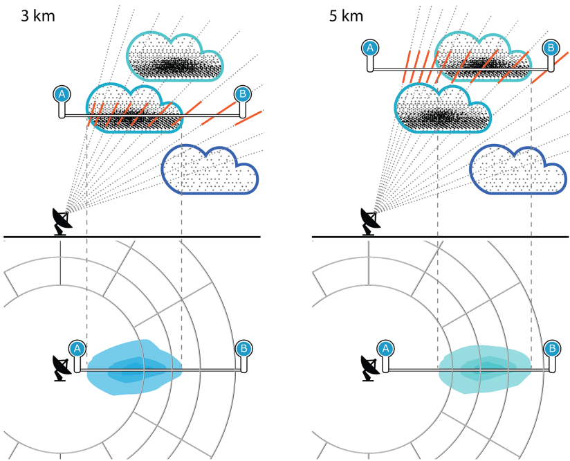
图 35 3 km 和 5 km 高度处的 CAPPI
