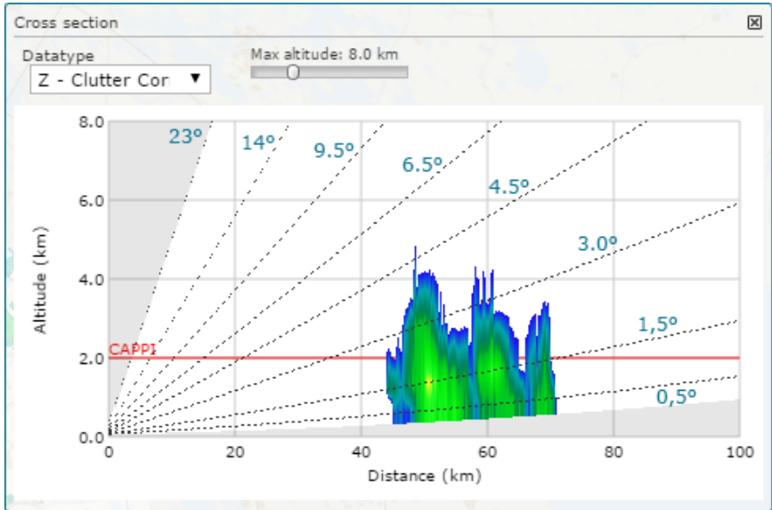
图 14 横截面工具, CAPPI 示例
