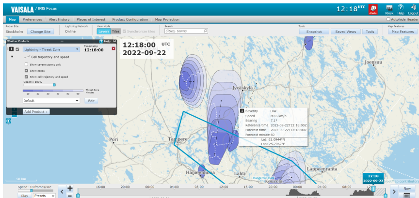
图 56 Lightning Threat Zone 产品。
