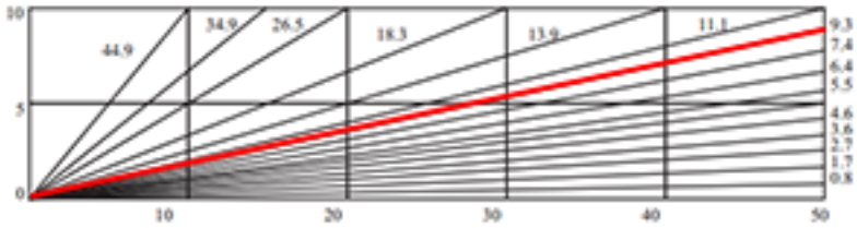
图 42 PPI 测量定义的仰角
