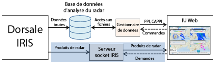
Figure 50 Flux de données de produits IRIS Analysis vers IRIS Focus
