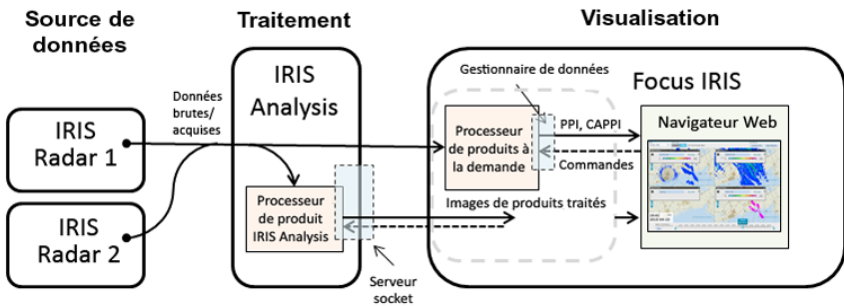
Figure 25 Flux de données IRIS Focus
