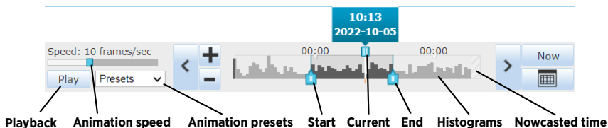
Рис. 8 Управление анимацией
