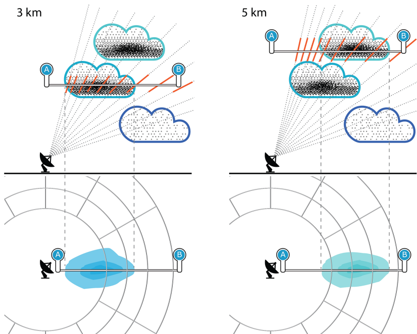
Рис. 35 CAPPI с высотой 3 и 5 км
