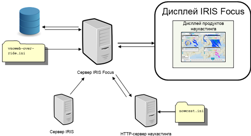
Рис. 18 Архитектура наукастинга
