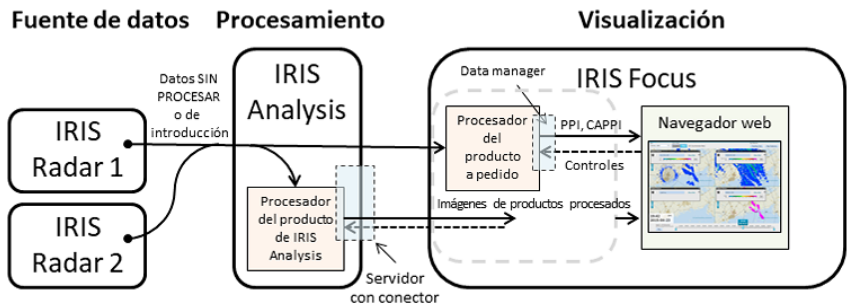
Figura 25 Flujo de datos de IRIS Focus
