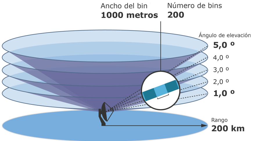
Figura 22 Bins y barridos
