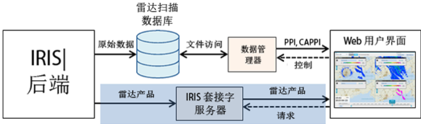
图 54 IRIS Analysis 到 IRIS Focus 的产品数据流
