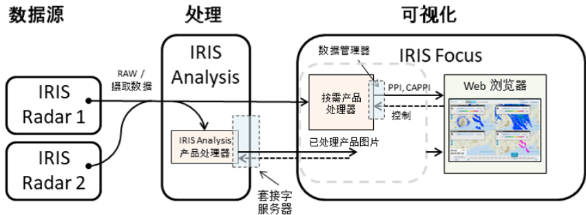
图 28 IRIS Focus 数据流
