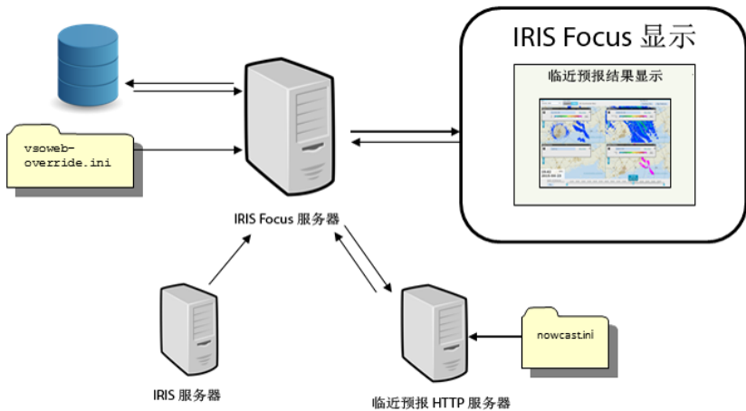
图 21 临近预报架构
