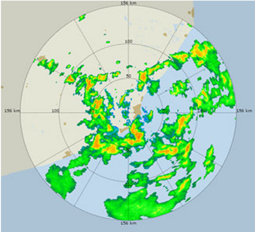
그림 14 강수 시 신호 반사율
