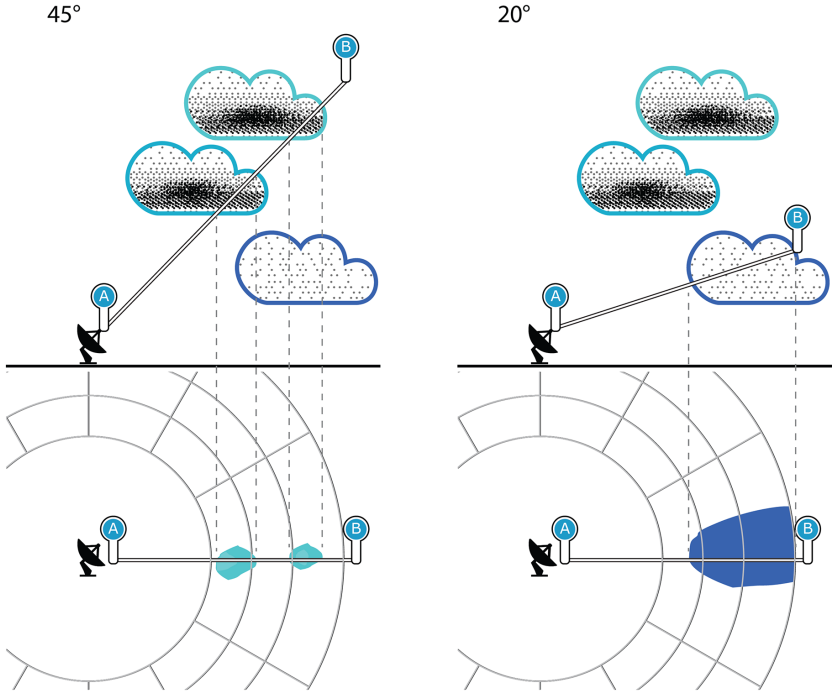
그림 42 45° 및 20° 양각의 PPI
