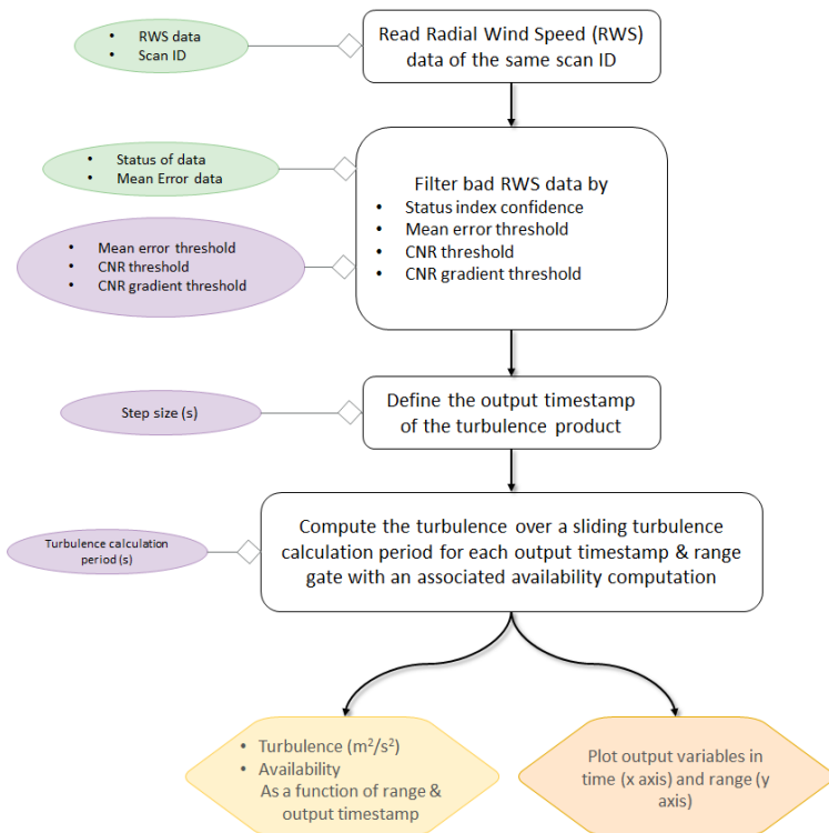
Рис. 52 Расчет турбулентности
