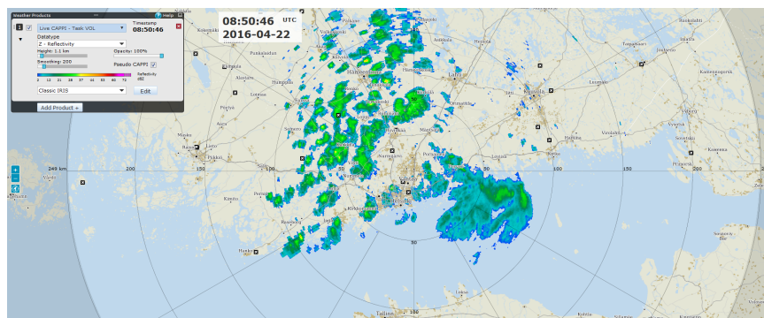
Рис. 32 Пример CAPPI
