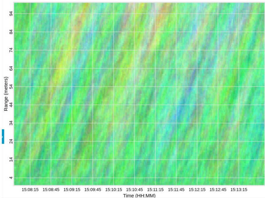
Рис. 53 Пример RTI
