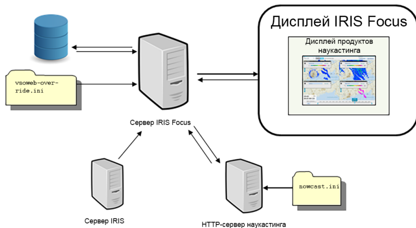
Рис. 21 Архитектура наукастинга
