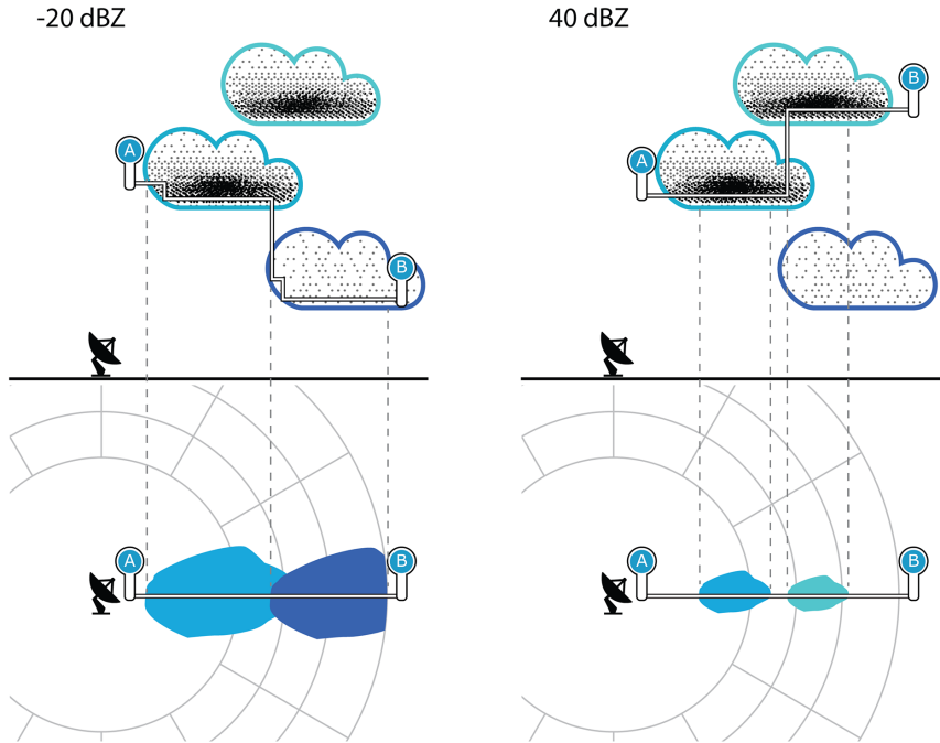
Рис. 31 BASE , пороговые значения -20 и 40 дБЗ
