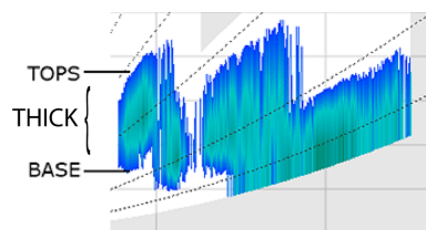
Рис. 44 THICK с BASE и TOPS
