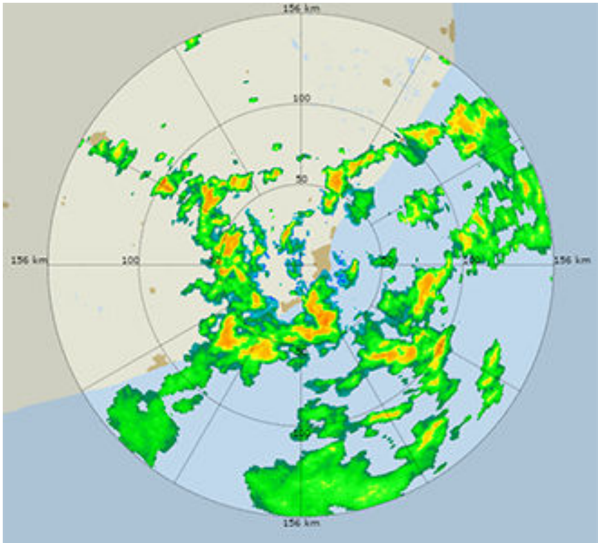
Рис. 14 Отражаемость сигнала при атмосферных осадках
