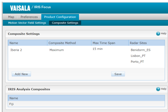
图 72 组合设置
