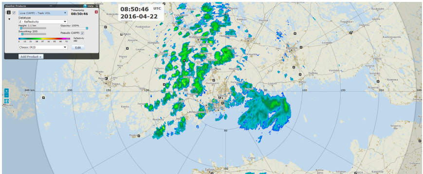
图 33 CAPPI 示例
