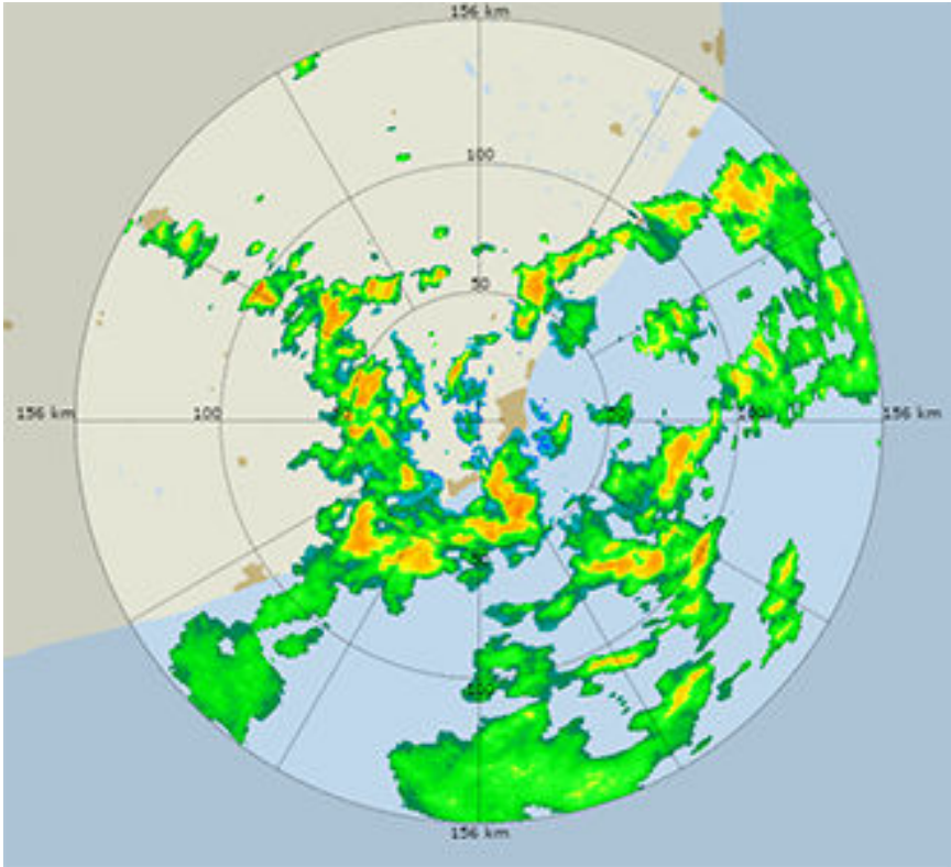
图 15 降水中的信号反射率
