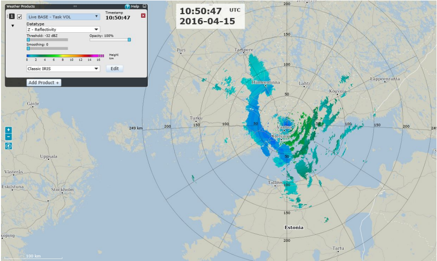
图 30 BASE 示例
