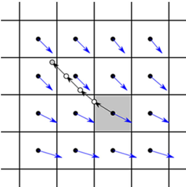
图 23 平流产品
