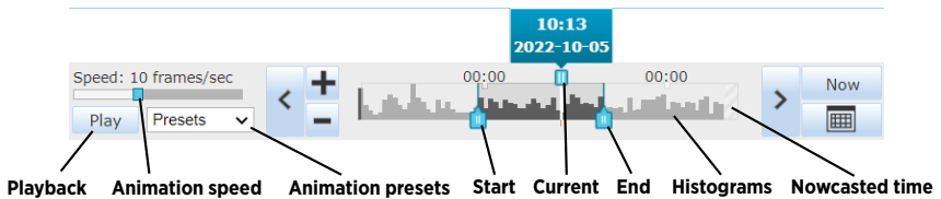
图 10 动画控件
