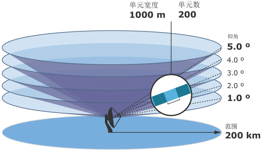
图 26 单元和扫描
