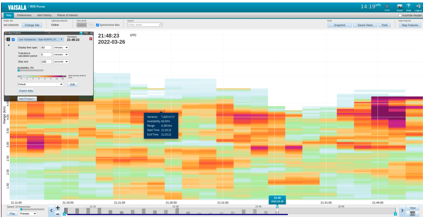
图 50 Turbulence 示例
