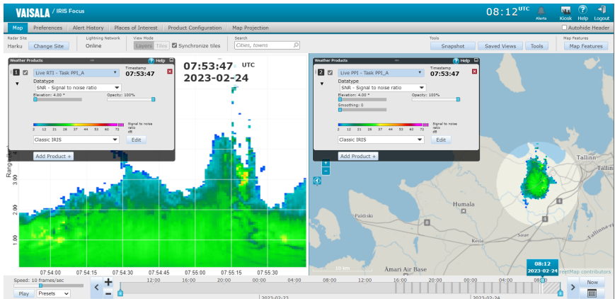
图 53 RTI 示例
