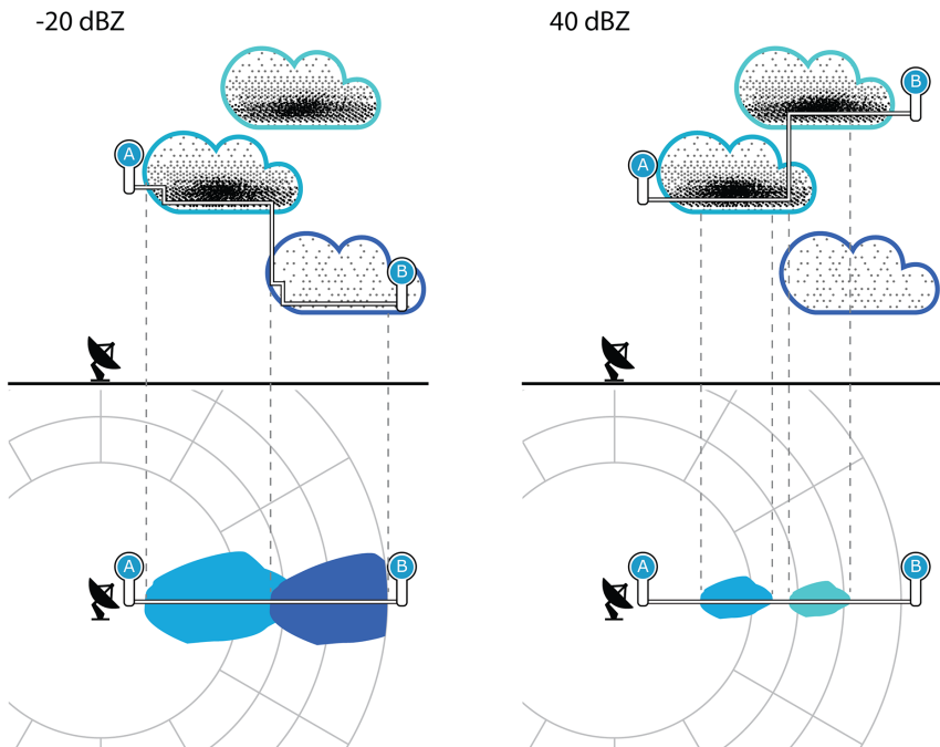
图 32 BASE，阈值为 -20 和 40 dBZ
