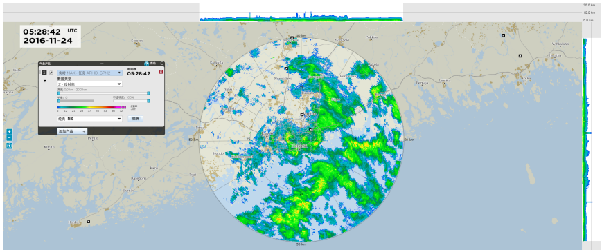
图 38 MAX 示例
