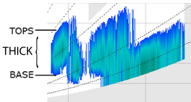
图 31 BASE 和 TOPS 产品
