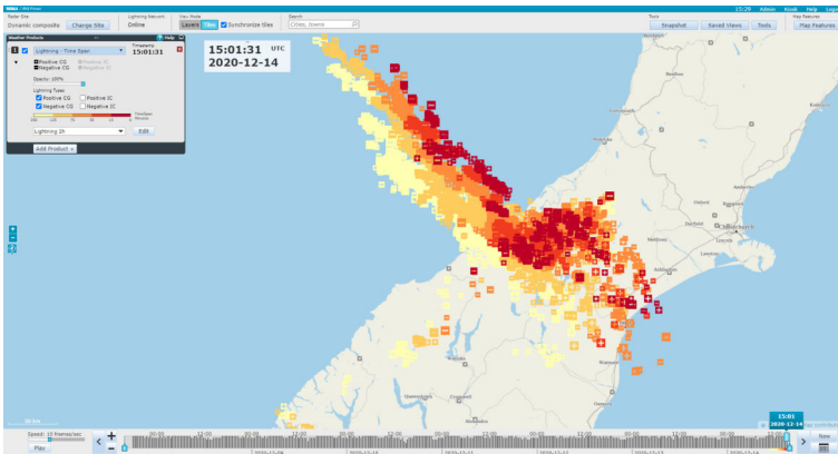
图 58 TimeSpan 产品
