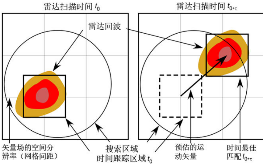
图 57 计算 TREC
