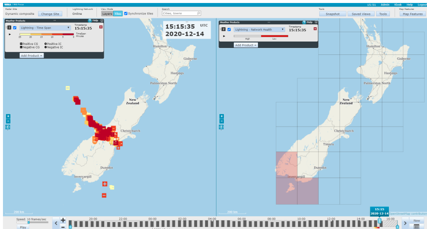
图 2 以平铺视图显示的闪电数据
