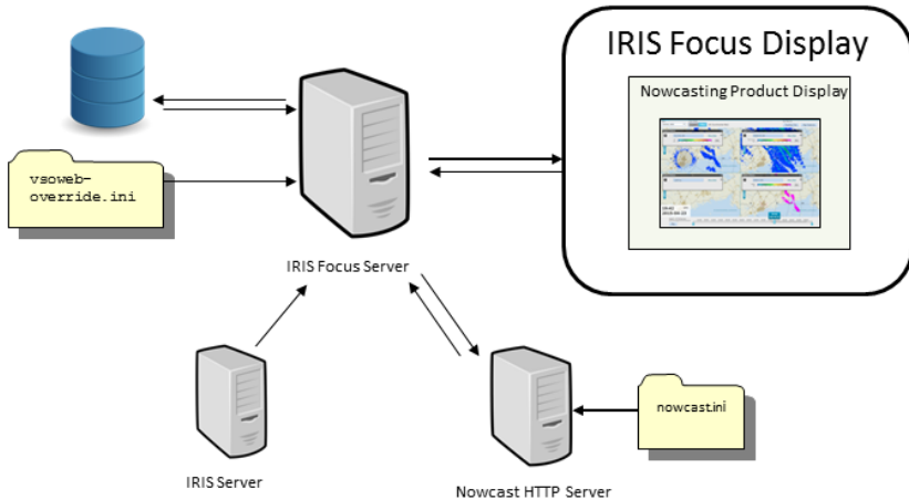
Figure 22 Architecture de la prévision immédiate
