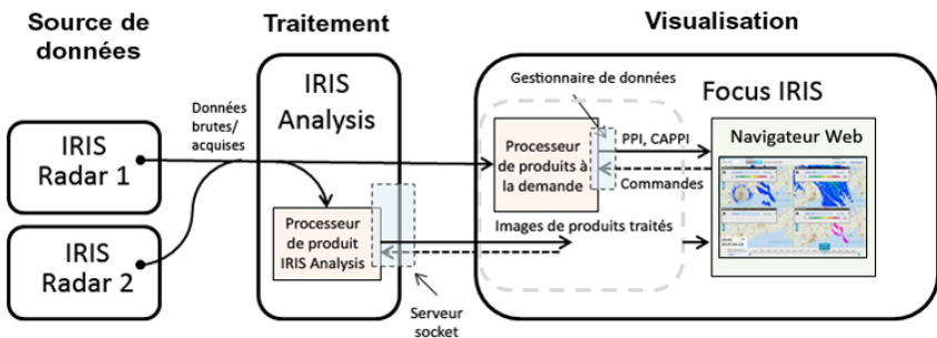
Figure 29 Flux de données IRIS Focus
