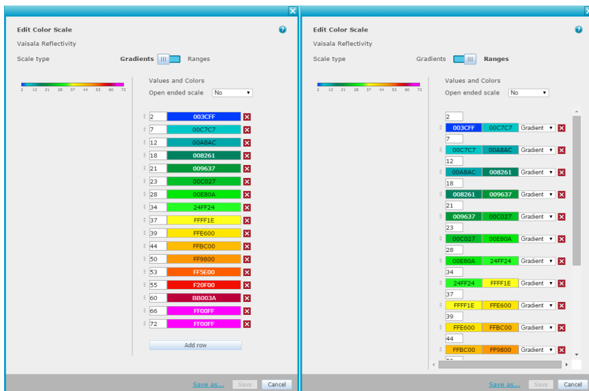
Рис. 16 Режимы редактора цветовой шкалы для продуктов радара
