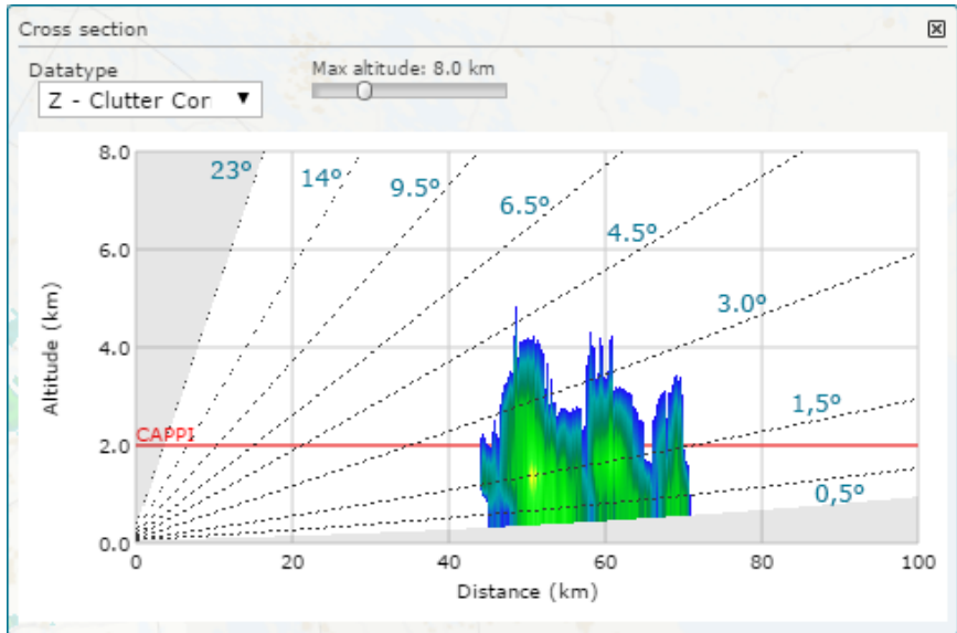
Рис. 13 Инструмент «Вертикальный разрез», пример САРР
