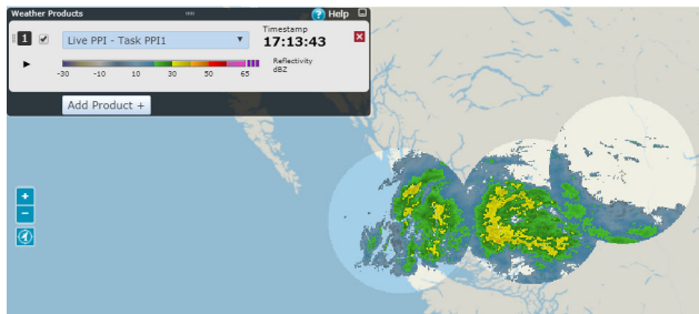
Рис. 20 Пример композита радара
