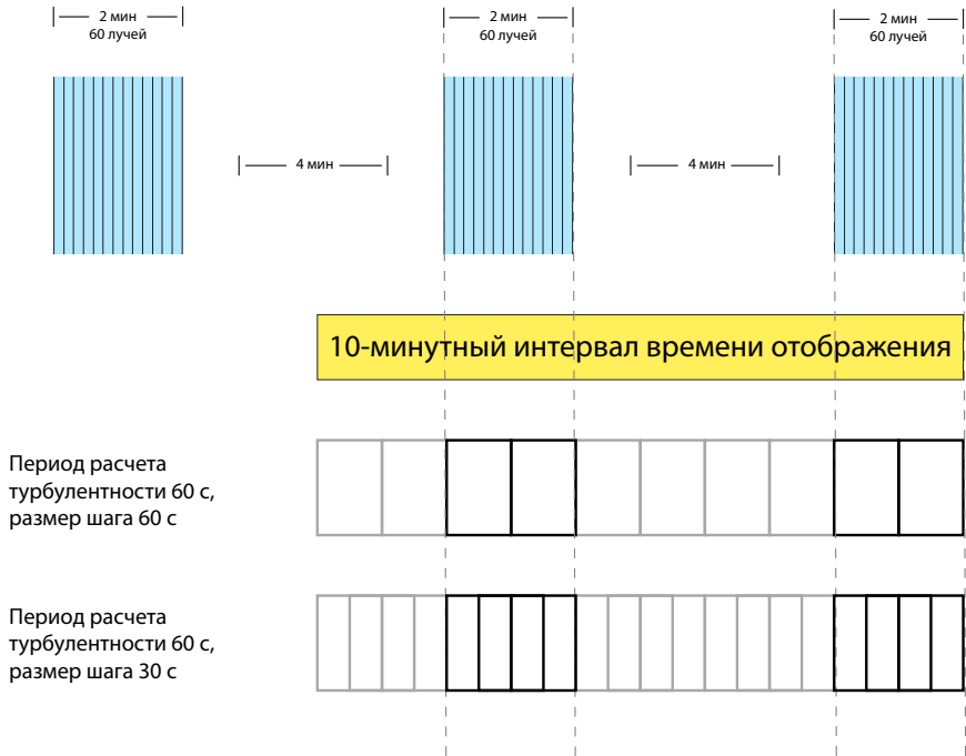
Рис. 51 Период расчета турбулентности и размер шага
