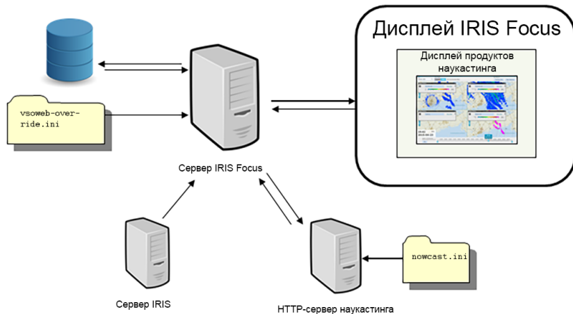
Рис. 22 Архитектура наукастинга
