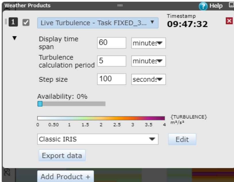
Рис. 52 Продукт Turbulence на панели Метеорологические производные
