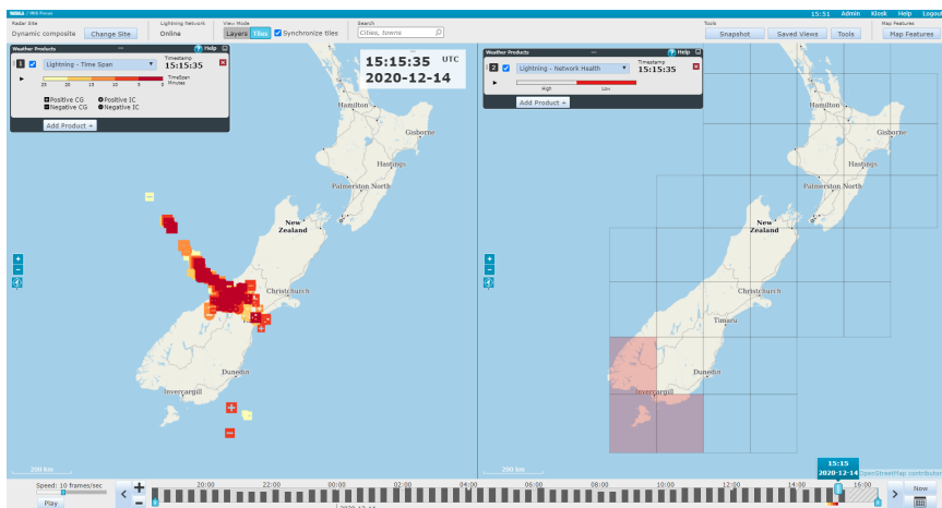
Рис. 2 Данные молний отображаются в виде плиток
