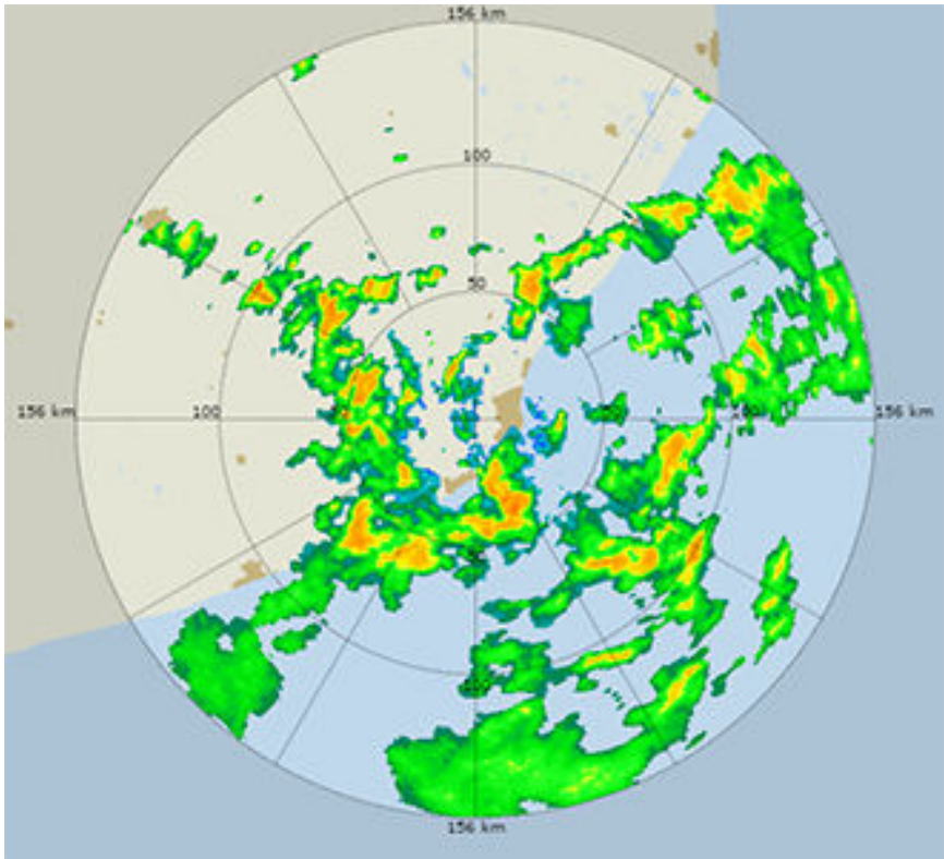
Рис. 15 Отражаемость сигнала при атмосферных осадках
