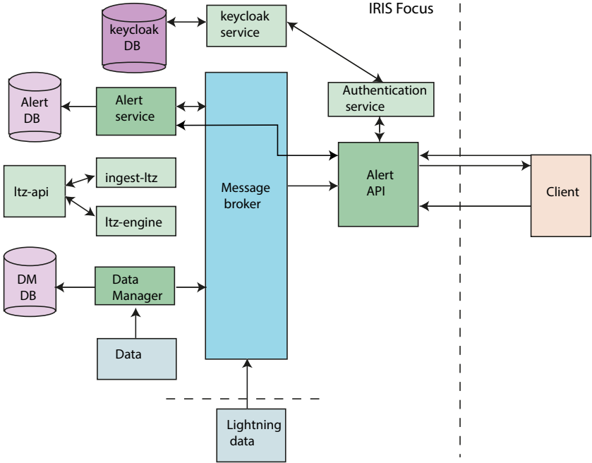
图 23 IRIS Focus 中的警报 API 架构
