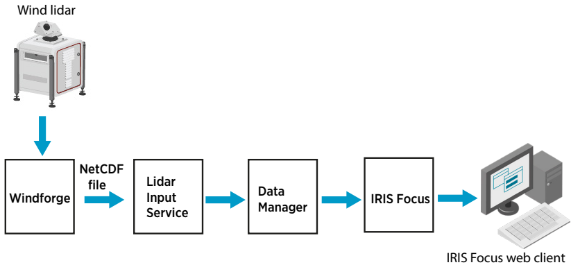
图 6 IRIS Focus 激光雷达架构
