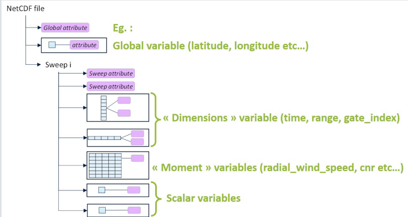
图 25 维萨拉 NetCDF 架构
