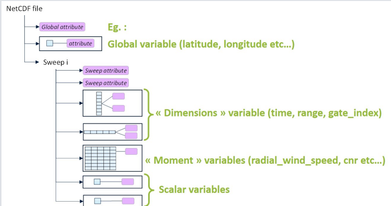
Рис. 25 Архитектура Vaisala netCDF
