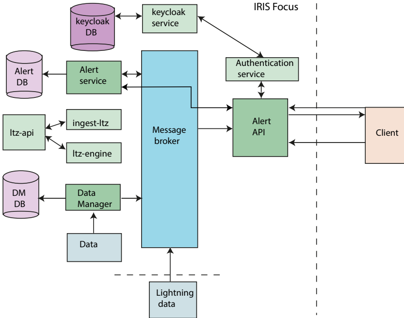
Figura 23 Arquitectura de API de alertas en IRIS Focus
