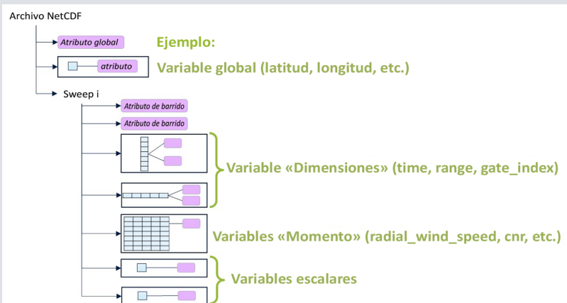
Figura 25 Arquitectura NetCDF de Vaisala
