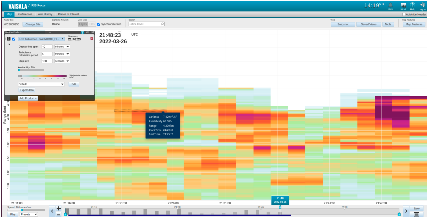
그림 47 Turbulence 예
