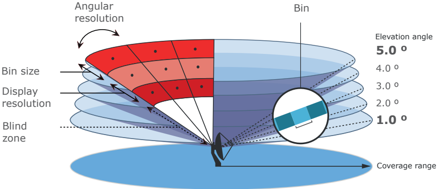
그림 24 장치 빔 전파
