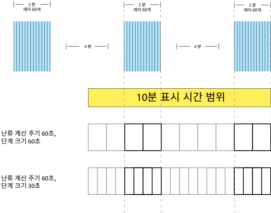
그림 48 난기류 계산 기간 및 단계 크기
