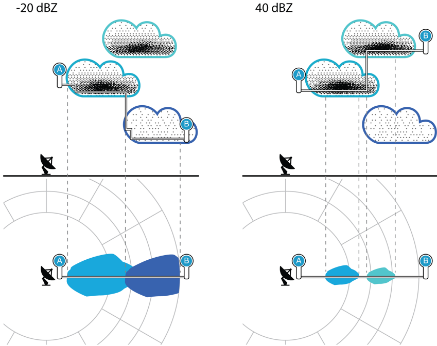
그림 29 BASE, -20 및 40dBZ 한계값
