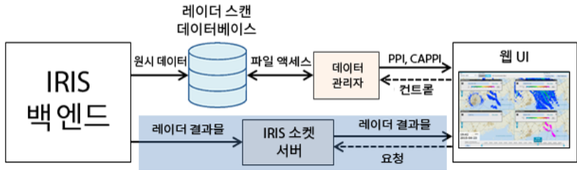
그림 51 IRIS Focus로의 IRIS Analysis 제품 데이터 흐름
