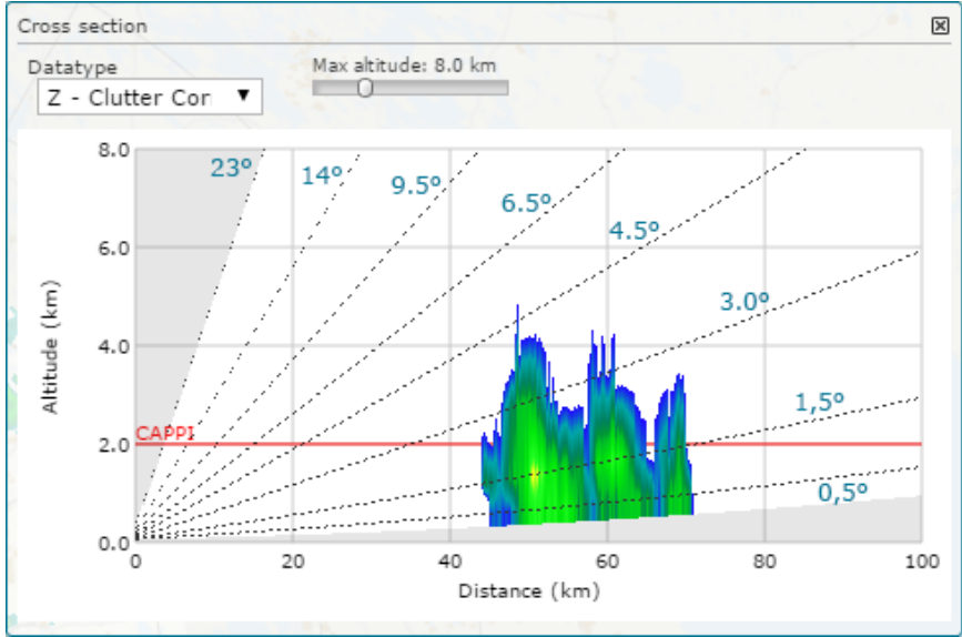
그림 11 단면 도구, CAPPI 예시
