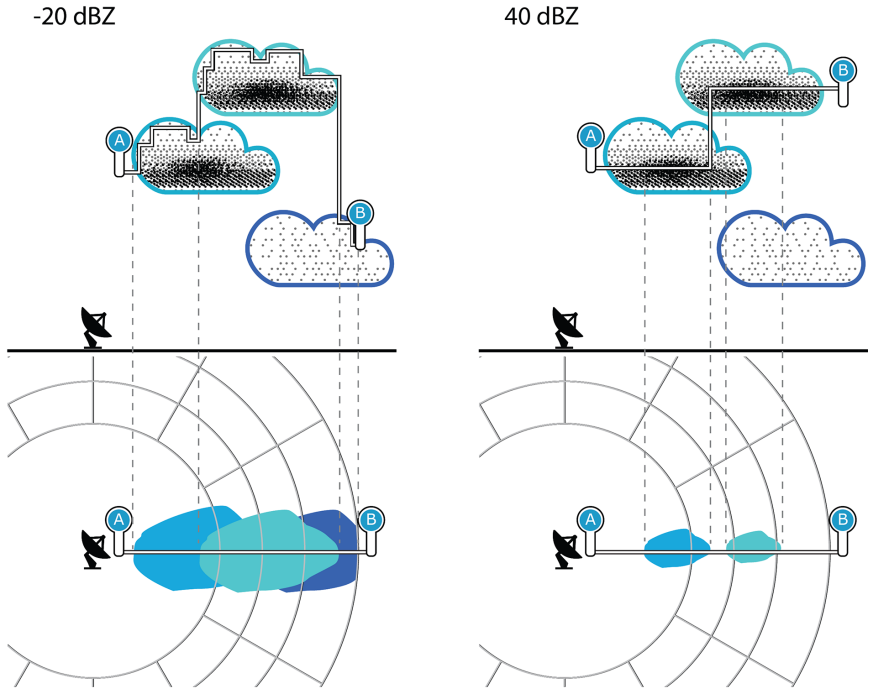
그림 46 TOPS , -20dBZ 및 40dBZ 한계값
