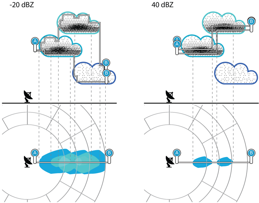
그림 43 THICK, -20dBZ 및 40dBZ 한계값
