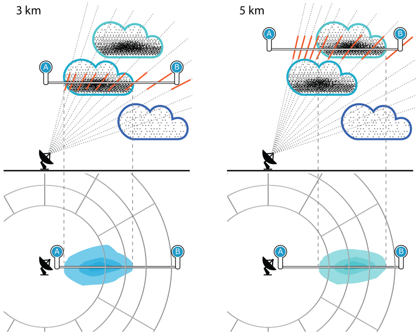
그림 32 CAPPI, 3km 및 5km 높이
