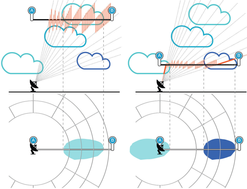
그림 33 Pseudo CAPPI 연장 CAPPI
