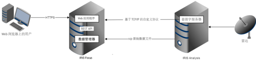
图 19 雷达数据传送路径
