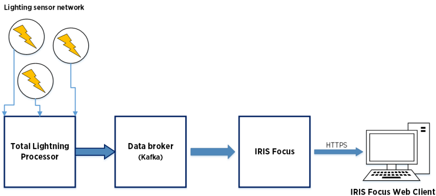
图 6 IRIS Focus 闪电体系结构
