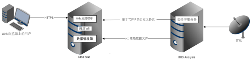
图 16 雷达数据传送路径
