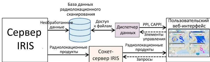
Рис. 5 Архитектура IRIS Focus для продуктов радаров
