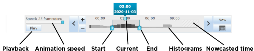
图 8 动画控件
