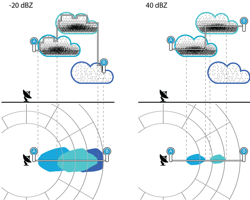
Figura 49 TOPS con umbrales de -20 dBZ y 40 dBZ
