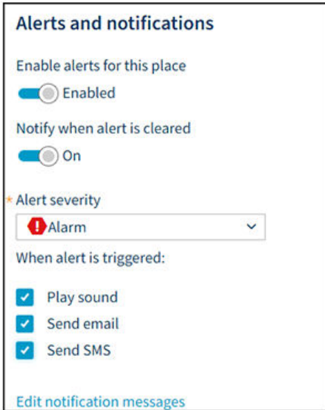
Figura 62 Configuración de notificaciones en la pestaña Área de interés
