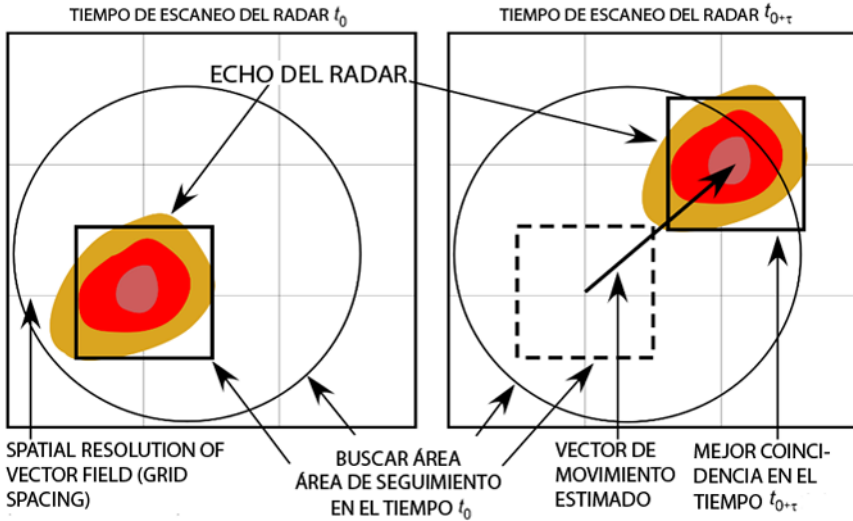
Figura 53 Cálculo de TREC
