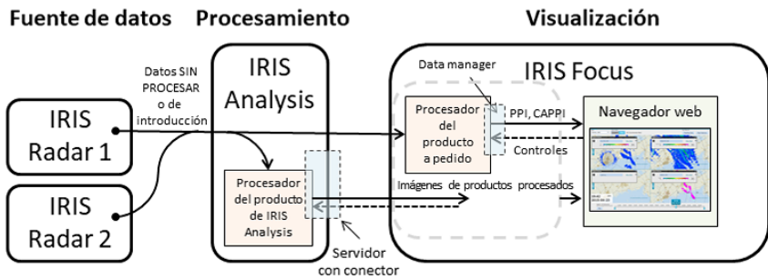
Figura 25 Flujo de datos de IRIS Focus
