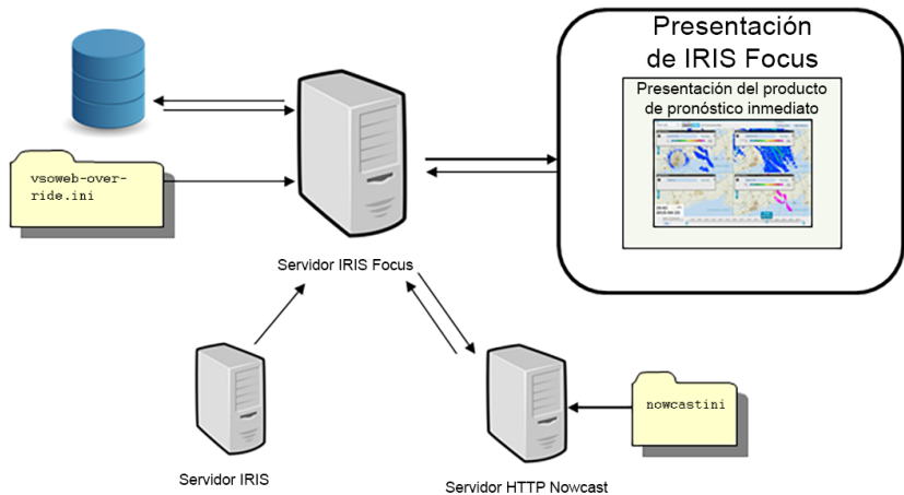
Figura 18 Arquitectura del pronóstico inmediato
